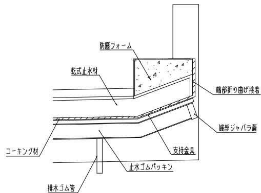
地覆部側面図
