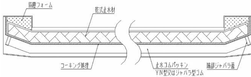
車道部断面図
